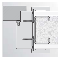
montáž na vruty do stěny ze sádkartónu
