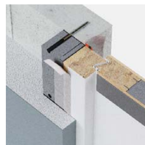
systém „pasivní“ (stojna)
