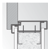
rohová zárubeň velká montáž na sádkartonovou stěnu
