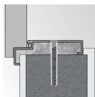
rohová zárubeň velká montáž pomocí šroubů
